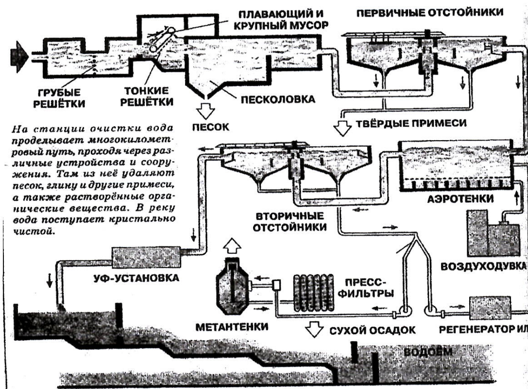
Рис. 2 - Схема очистного сооружения
